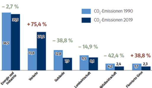
Die Grafik zeigt die Entwicklung der Treibhausgasemissionen von 1990 bis 2019 in Österreich, in Mio. t CO 2 -Äquivalente. © Salzburger Bauer, Quelle: Umweltbundesamt, Daten Juli 2020
