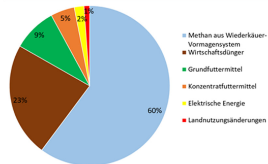
Treibhausgasemissionsquellen aus der Milcherzeugung in Österreich. 60 % stammen aus der verdauungsbedingten Methanemission, weitere 23 % trägt die Wirtschaftsdüngerlagerungs- und Ausbringung bei, 9 % Grundfuttermittel und 5% Konzentratfuttermittel.
