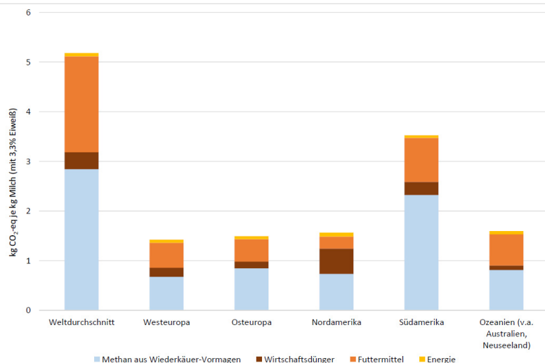
Die Grafik zeigt die THG-Emissionen der globalen Milcherzeugung auf Basis 3,3 % Eiweiß. Die europäische Milchproduktion schneidet diesbezüglich am besten ab. 1 kg Milch verursacht in Westeuropa 1,42 kg CO 2 -Äquivalente, in Osteuropa 1,49, weltweit liegt der Durchschnitt bei 5,18 kg CO 2 -Äquivalente. © BOKU/Hörtenhuber (2020) nach Gerber et al. (2017)
